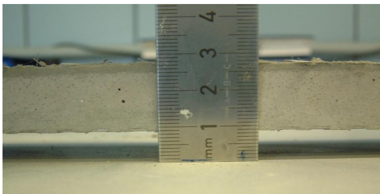
Figura 4 – Misura della convessità di una malta espansiva
