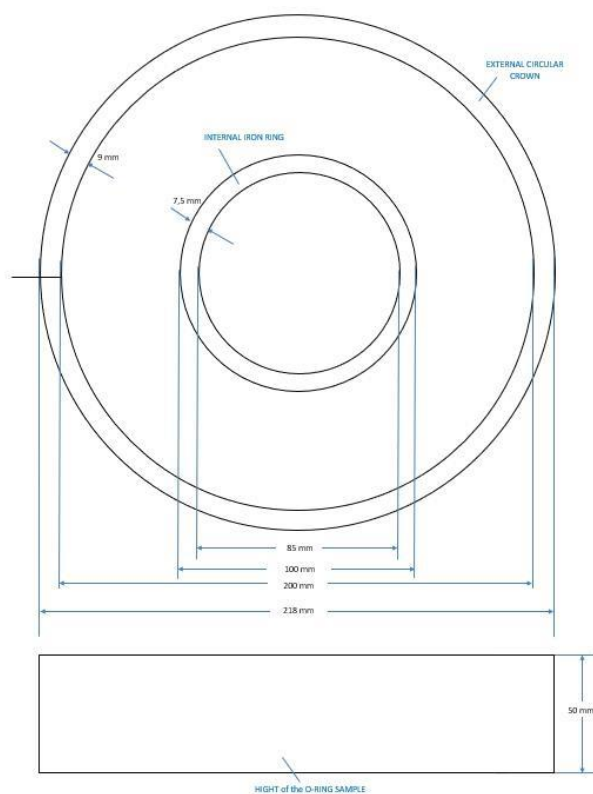
Figura 4 – Dimensioni della cassaforma per O-Ring test
